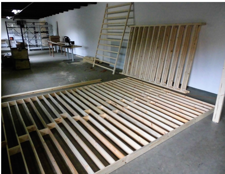
Fanereol og skillevæg, klar til opsætning
